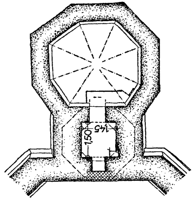
④ GRUNDRISS ÜBER +0,46 m.
