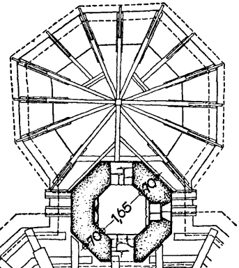
GRUNDRISS ÜBER +0,63 m.
