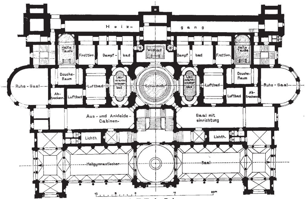
Abb. 1. Friedrichsbad in Baden. Hauptgeschoß.
