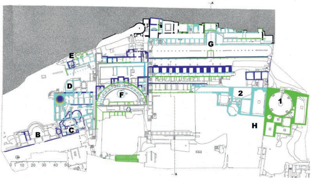
Abb. 6: Zweite Phase der Baugenesse der Gebäudestrukturen innerhalb des Archäologischen Parks von Baiae. Die Gebäudebereiche sind entsprechend der Abbildungen 2 und 3 mit den Buchstaben B–H versehen. Im Sektor des Merkur (= Buchstabe H) befindet sich das augusteische Badegebäude (grün hervorgehoben) mit der Nummer 1; etwas später (1. Jh. n. Chr.) folgt das Badegebäude (in cyan) Nr. 2. (Quelle: Mariarosaria Borriello/Antonio d’Ambrosio, Baiae – Misenum, in: Forma Italia, Regio I, Bd. 14, Florenz 1979, Tav. I, Pianta a Quota: 37,7 m; Vorläufige Phaseinteilung: M. Nieberle).
