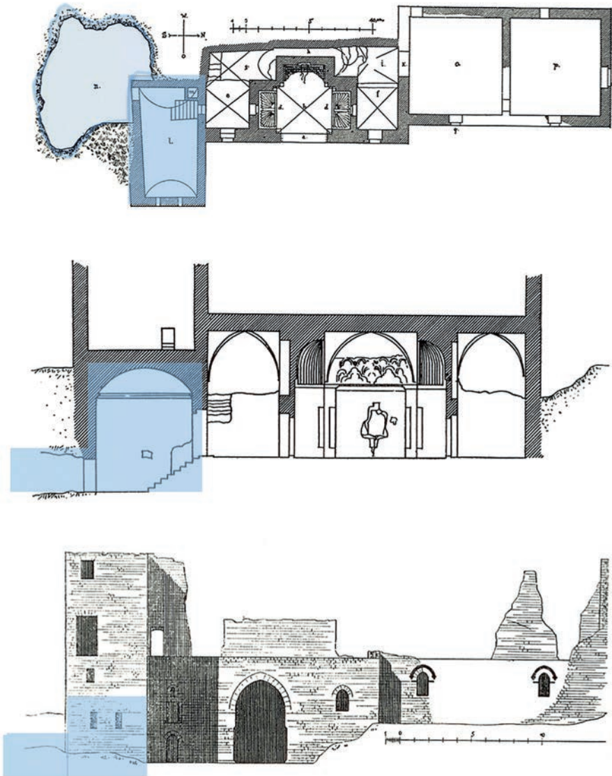
Abb. 19: Grundriss, Querschnitt und Aufsicht des Uscibene, um 1150 (Quelle: Adolf Goldschmidt, „Die normannischen Königspaläste in Palermo“, in: Zeitschrift für das Bauwesen 48 (1898), Abb. 5, 2, 1, mit Markierungen des Autors).
