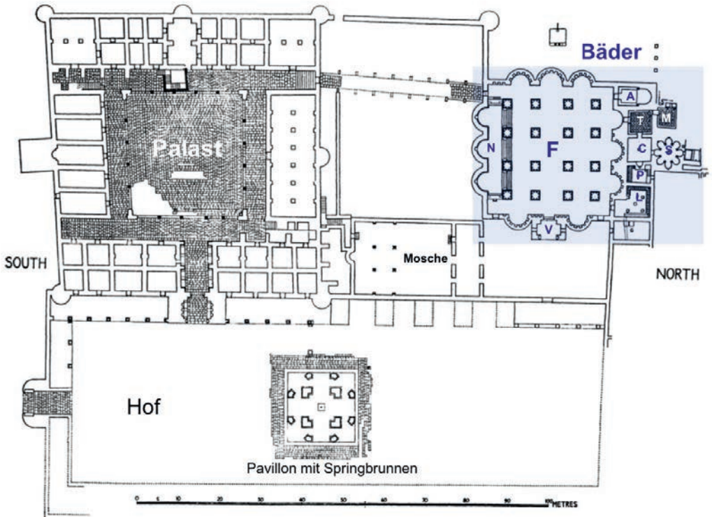
Abb. II: Grundrissplan des Palastes von Khirbat al-Mafjar (oder des Hisham), um 724–743 (Quelle: Robert H. Hamilton, Khirbat al-Mafjar. An Arabian Mansion in the Jordan Valley , Oxford 1959, Taf. 109, mit Beschriftungen und Markierungen des Autors).
