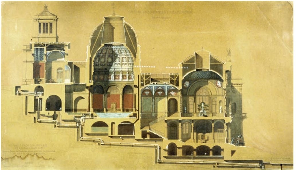
Abb. 25: Friedrichsbad in Baden-Baden, Querschnitt. Die großformatige Darstellung von 1881 basiert auf der Bauaufnahme eines Baupraktikanten (GLA Karlsruhe 424 K Baden-Baden 006/3.001).
