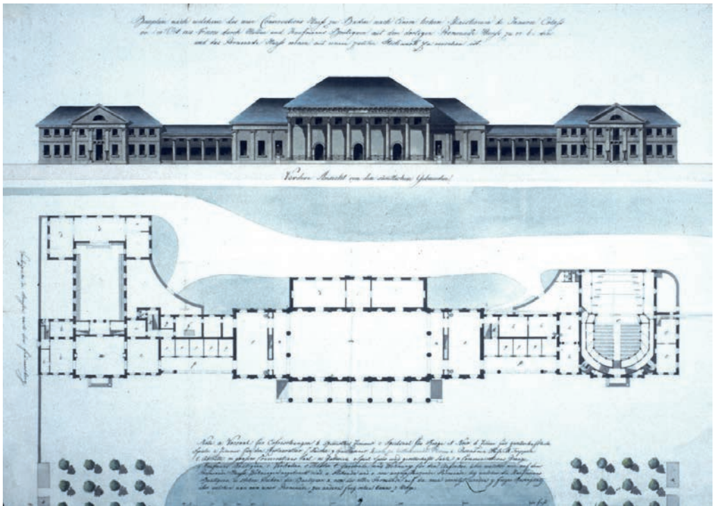
Abb. 9: Kurhaus in Baden-Baden (originaler Entwurf), Architekt Friedrich Weinbrenner (1822–24) General-landesarchiv Karlsruhe G Baupläne Baden-Baden 116.
